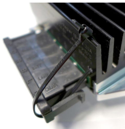
Zugentlastung des Kombisteckers mit einem Kabelbinder
